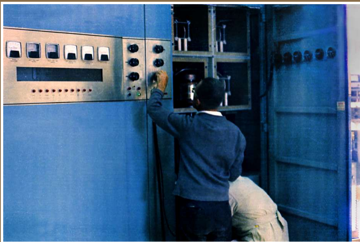
Fig. 25. Instalación de estación de 50 mil watts de potencia de Radio Educación, finales de los años sesenta. Acervo de Ignacio Espinosa.
